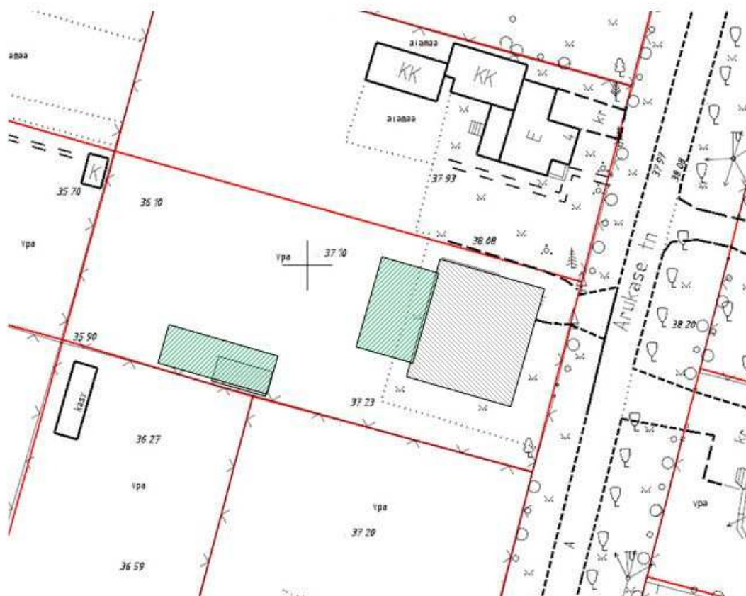
LISA 1 – TINGLIKU EHITUSALA SKEEM
